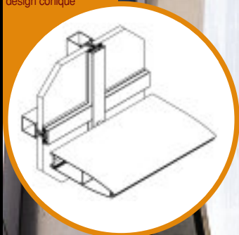
BRISE SOLEIL AA120 KALUMEN 270 mm de profondeur design conique
