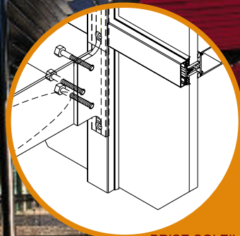
BRISE SOLEIL AA120 KALUMEN 800 mm de profondeur design aile d'avion
