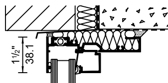
FENÊTRE INCORPORANT LA MÉTHODE DE L'ÉCRAN DE PLUIE
