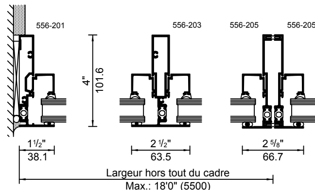
1 JAMBAGE 2 MENEAU TUBULAIRE 3 MENEAU JUMELÉ MULTI-MODULAIRE
