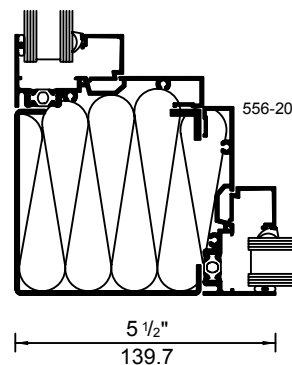
COIN EXTÉRIEUR DE 90°
