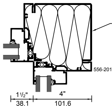
COIN INTÉRIEUR DE 90°
