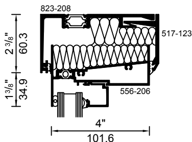
FENÊTRE INCORPORANT LA MÉTHODE DE L'ÉCRAN DE PLUIE
