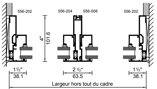
1 JAMBAGE 2 MENEAU JUMELÉ 3 JAMBAGE
