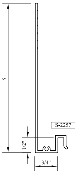
"E1" HEAD/JAMB PANNING E1
