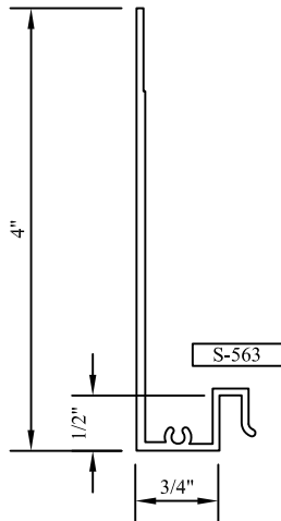
"E" MODIFIED HEAD/JAMB PANNING EM
