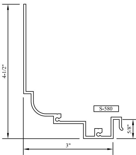
"Y" HEAD/JAMB PANNING Y
