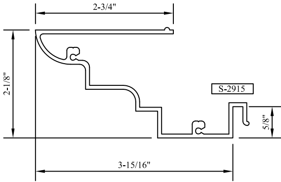
"A4" HEAD/JAMB PANNING A4
