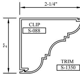
#25 TRIM & #9 CLIP
