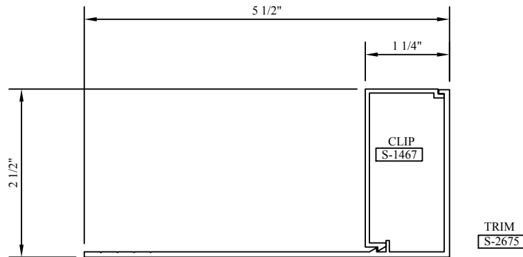
#70 TRIM & #70 CLIP
