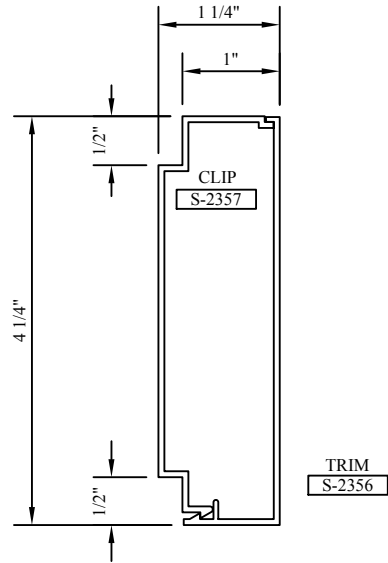
#59 TRIM & #59 CLIP
