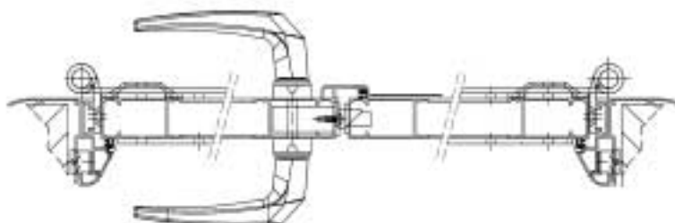
Volet 2 vantaux avec penture et contre penture. Dormant de pose et béquille double avec serrure à clef
