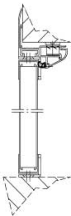
Volet plein 1 vantail avec dormant de pose 3 côtés
