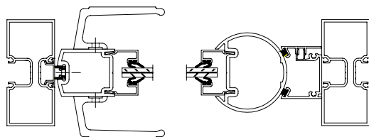
Porte K190 grand trafic avec assemblage par soudure sous argon et toiles d'aluminium de 3,5 à 4 mm d'épaisseur.
