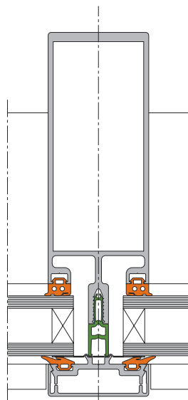
Schnitt der Fassade AA 100
